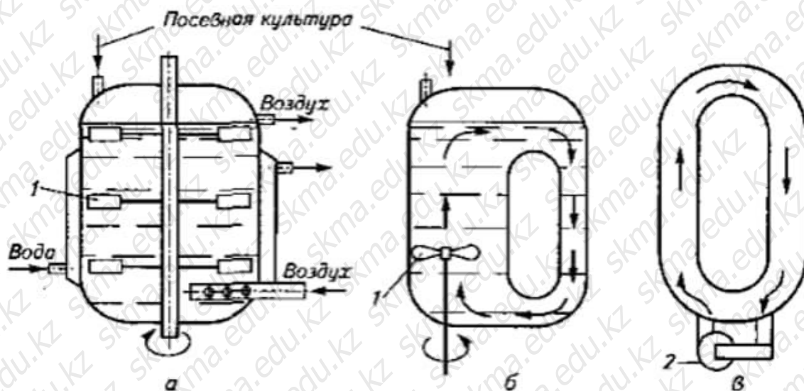
Рисунок 3. Схемы ферменторов.
