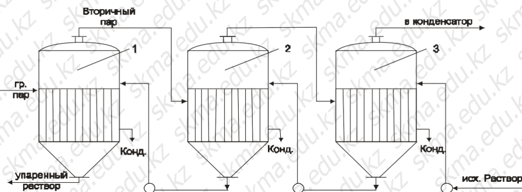
Рис. 13.3 Многокорпусная прямоточная вакуум-выпарная установка
