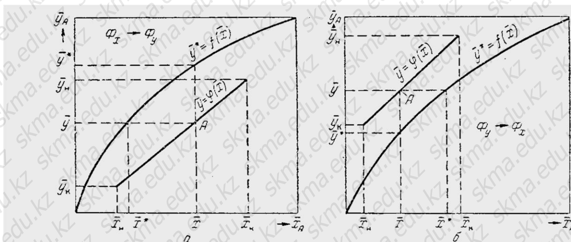
Рис. 14.3 Определение направления массопередаче по у-х-диаграмме:
